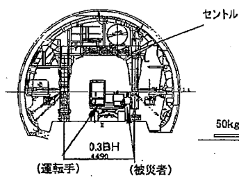
断面図(切羽より見て)
